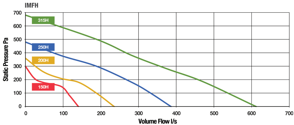
IMF Mixed Flow Arctic Fan
